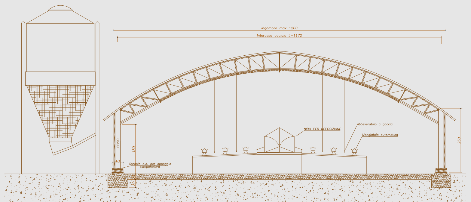
TUNNEL RETICOLARE PER OVAIOLE
